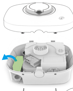
TX10 Tornillo Torx M3x16mm x2
